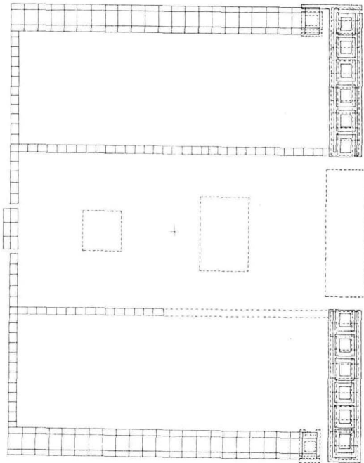
圖22. 皇龍寺 創建伽藍 配置圖
