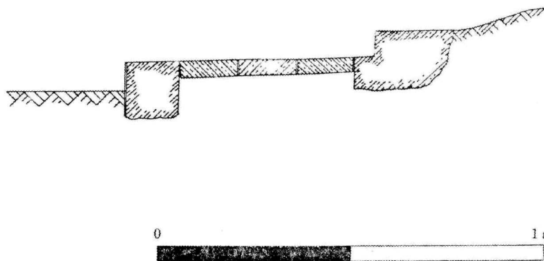
圖 5. 高仙寺 金堂 基壇石 實測圖
