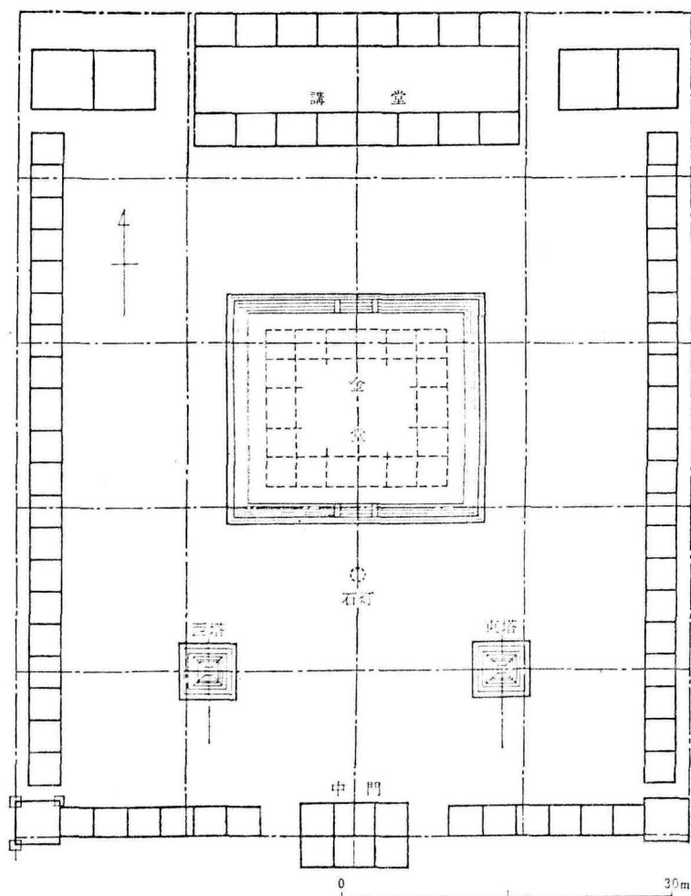
圖19. 千軍里 廢寺 伽藍 復元圖
