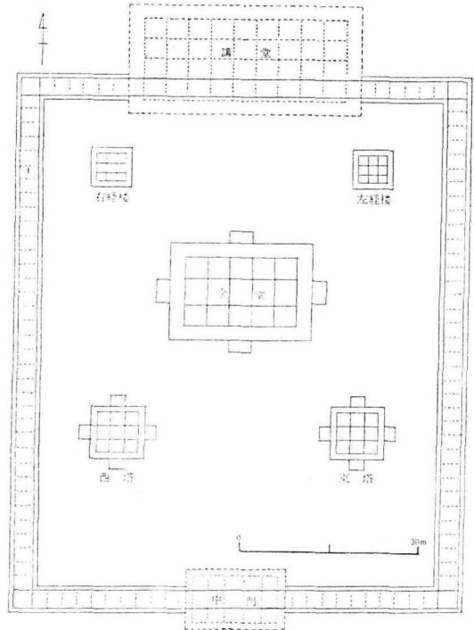
圖23. 四天王寺 伽藍 復元圖
