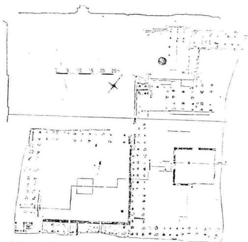
圖18. 高仙寺 伽藍 平面圖
