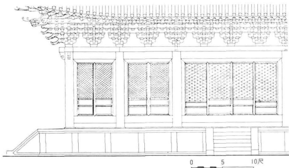
圖 7. 佛國寺 大雄殿 基壇立面圖
