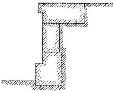
圖13. 高仙寺 講堂 基壇石 實測圖
