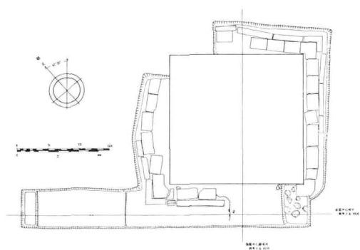
圖 9. 感恩寺 西塔 塔區
