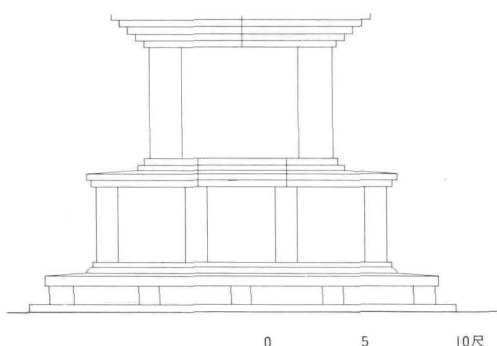
圖 8. 感恩寺 西塔基壇立面圖
