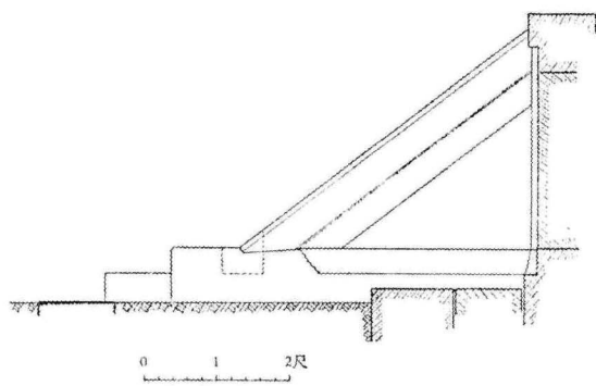
圖 4. 感恩寺 金堂 石階 推定 復原圖
