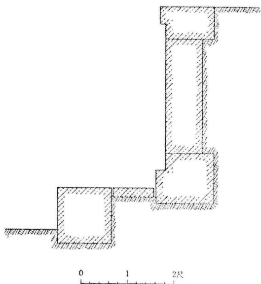
圖 3. 感恩寺 金堂 基壇石 復原圖
