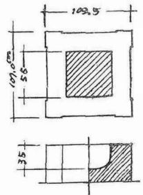
一層屋身舍利孔
