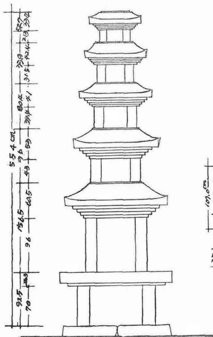
元敦岩莊所在 五層石塔 S = 1/40
